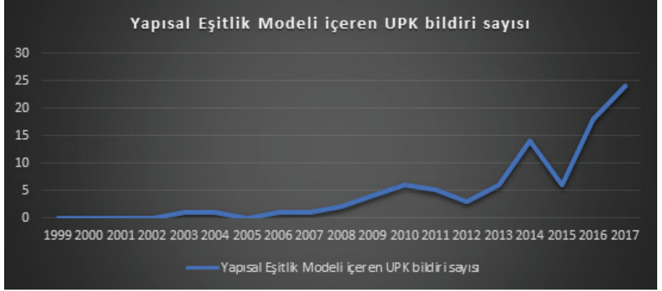
Şekil 3: 1999-2017 yılları arası ulusal pazarlama kongresi bildiri kitapçıklarında yer alan YEM analizi içeren bildirilerin yıllara göre değişimi
