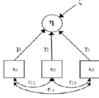
Oluşturuıcı ölçüm modeli (formative)
