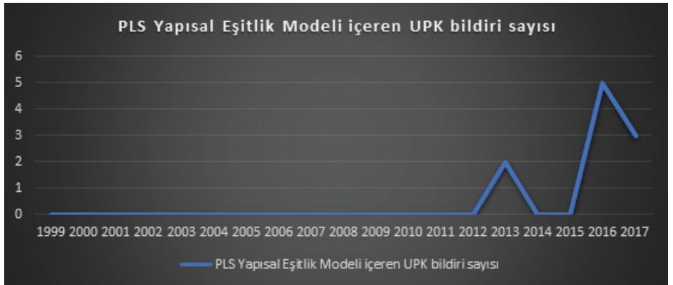
Şekil 4: 1999-2017 yılları arası ulusal pazarlama kongresi bildiri kitapçıklarında yer alan PLS-YEM analizi içeren bildirilerin yıllara göre değişimi
