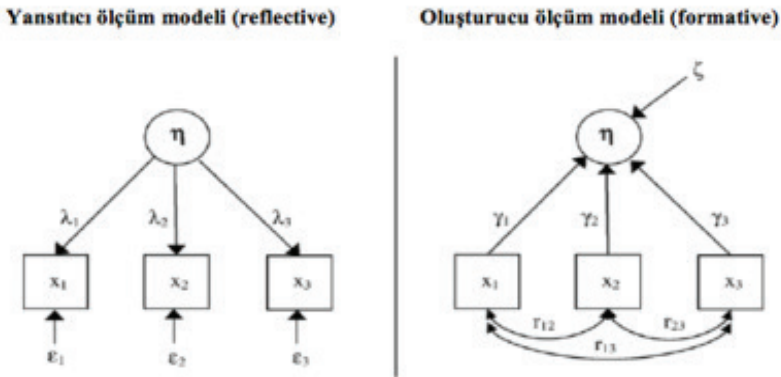
Şekil 6: Yansıtıcı ve oluşturuıcı ölçüm modeli
